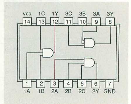
図5 LS11端子表
